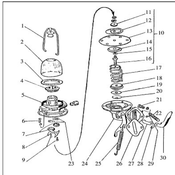
Hình 2.2. Các chi tiết của bơm xăng
