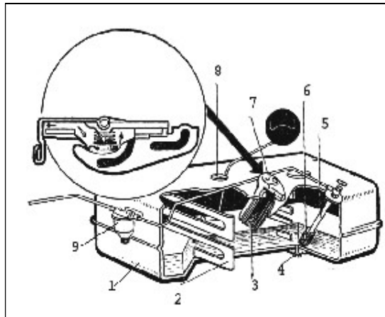
Hình 1.15. Cấu tạo thùng xăng
