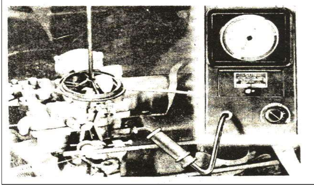
Hình 3.49. Kiểm tra bơm tăng tốc
