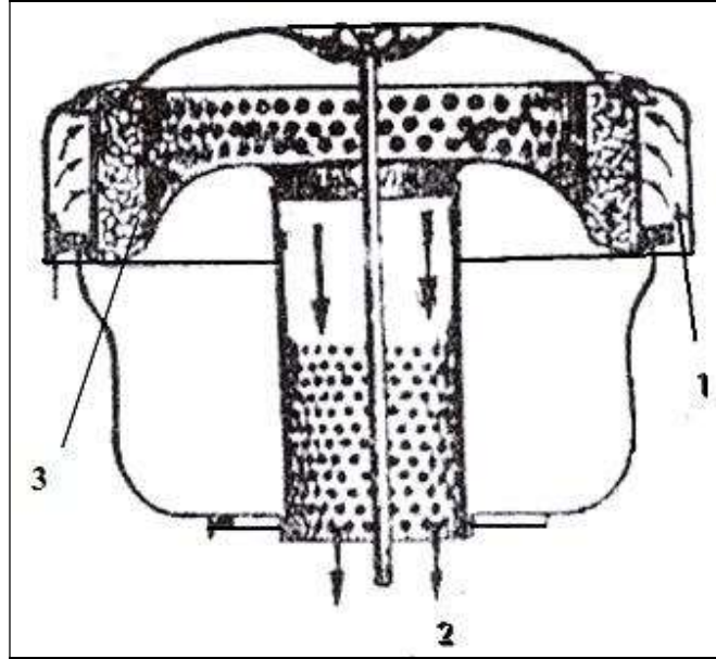
Hình 1.7. Cấu tạo bầu lọc khô
