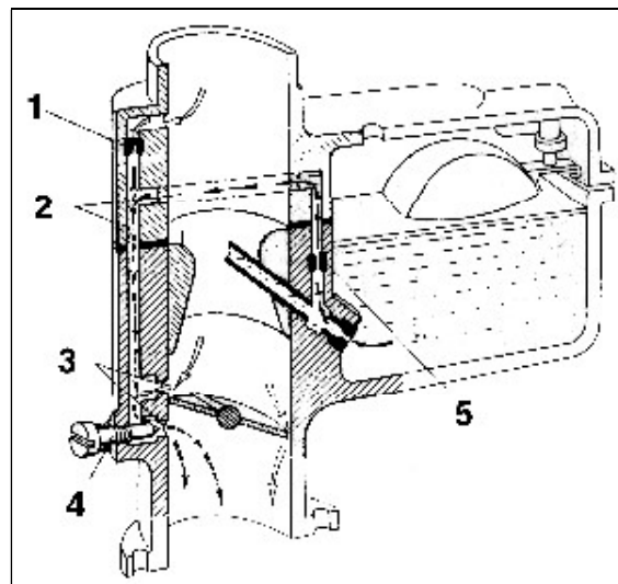
Hình 3.5. Hệ thống không tải
