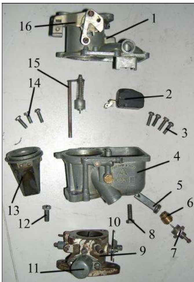
Hình 3.21. Các chi tiết và cụm chi tiết của bộ chế hoà khí
