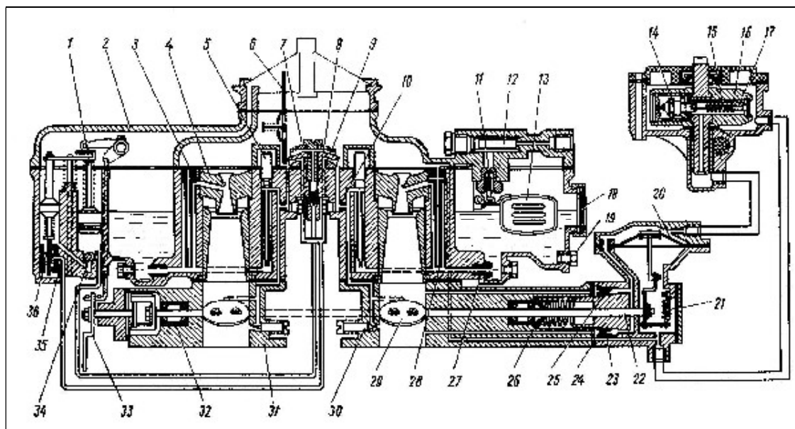
Hình 3.11. Bộ chế hòa khí - K126B
