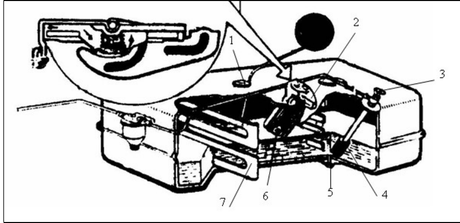
Hình 1.3. Thùng nhiên liệu
