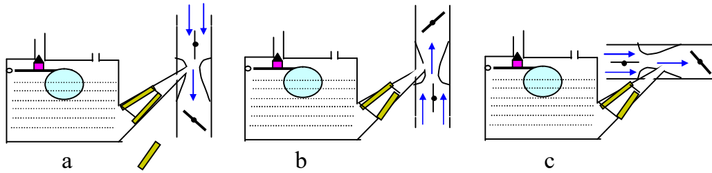
Hình 3.1. Sơ đồ chế hoà khí hút
