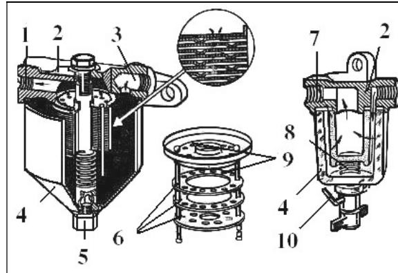
Hình 1.5. Bầu lọc nhiên liệu
