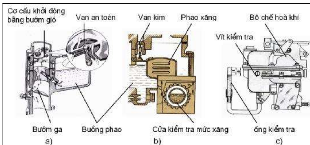
Hình 3.17. Kiểm tra mức xăng trong buồng phao
