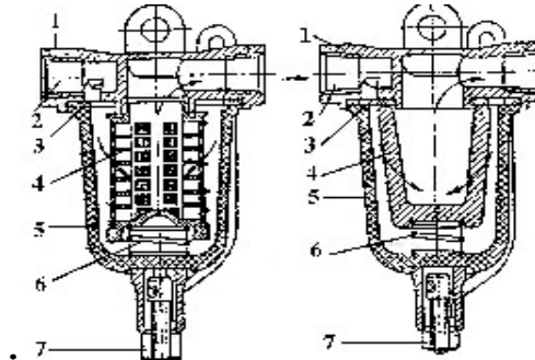
Hình 1.17. Bàu lọc nhiên liệu tinh
