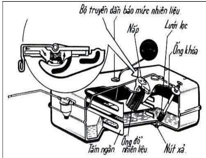
Hình 4.1. Thùng nhiên liệu
