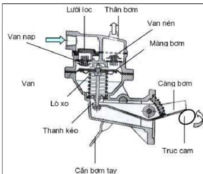
Hình 3.14. Sơ đồ cấu tạo bơm xăng
