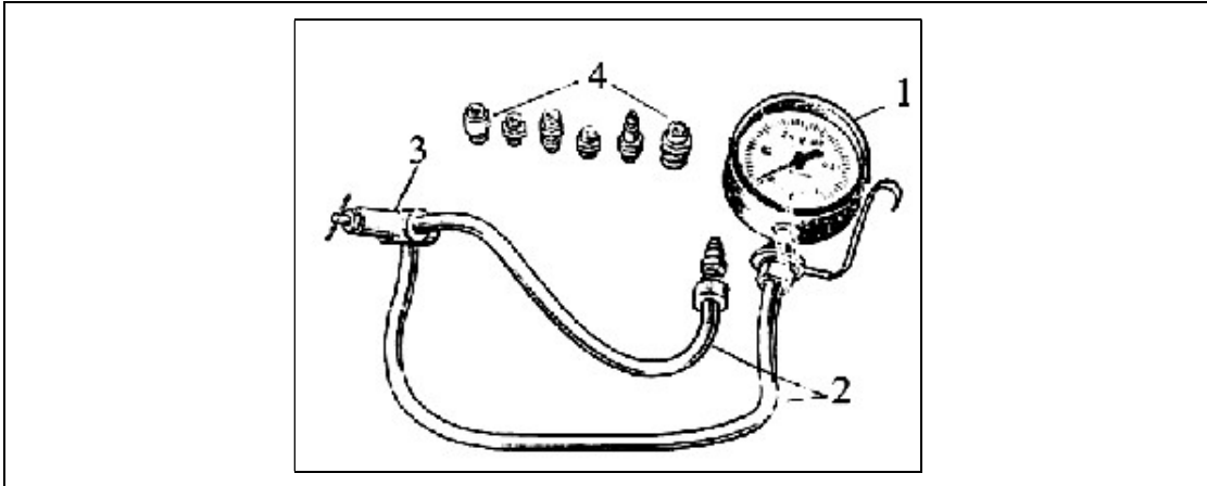
Hình 5.1. Thiết bị kiểm tra áp suất
