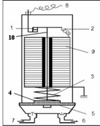
Hình 1.14. Bơm xăng điện kiểu màng
