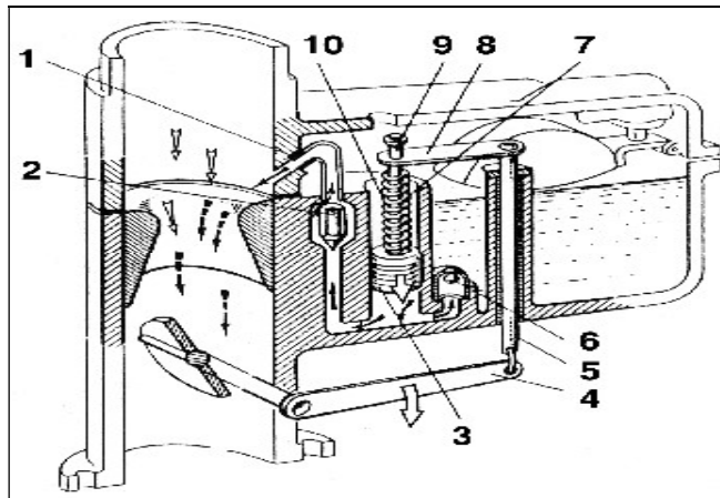
Hình 3.49. Hệ thống tăng tốc
