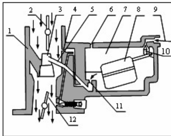
Hình 3.37. Hệ thống phun chính
