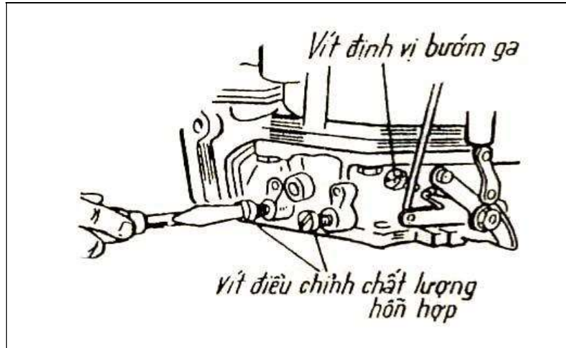
Hình 3.35. Điều chỉnh chế độ chạy không tải
