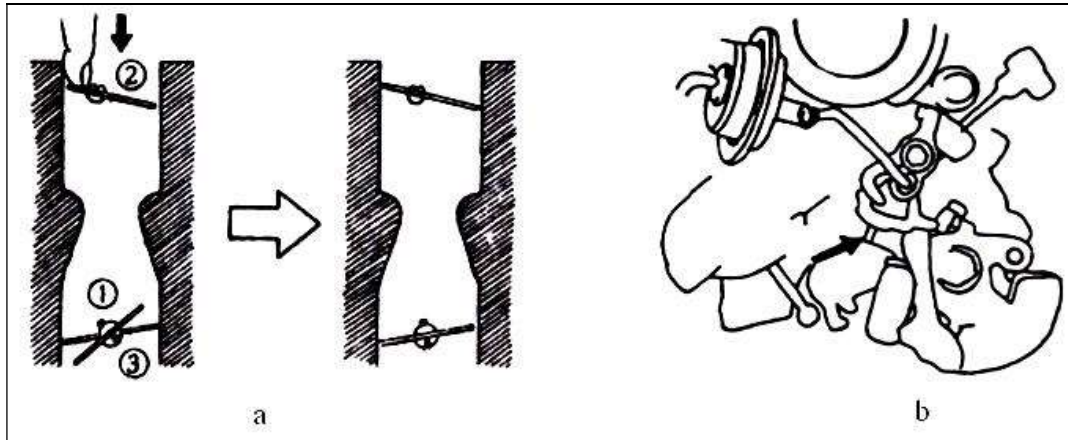
Hình 3.24. Điều chỉnh vòng quay không tải nhanh
