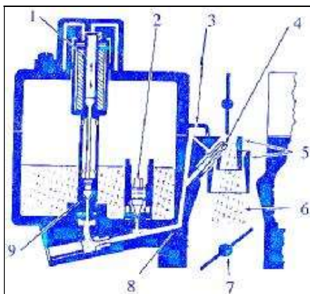
Hình 3.39. Cơ cấu điện từ điều khiển kim gicơ chính
