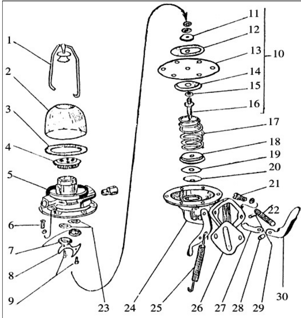
Hình 5.3. Các chi tiết của bơm xăng
