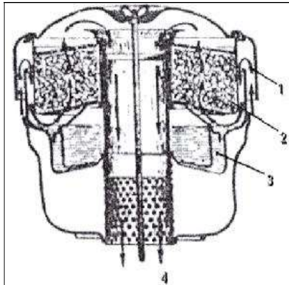
Hình 1.8. Cấu tạo bầu lọc ướt
