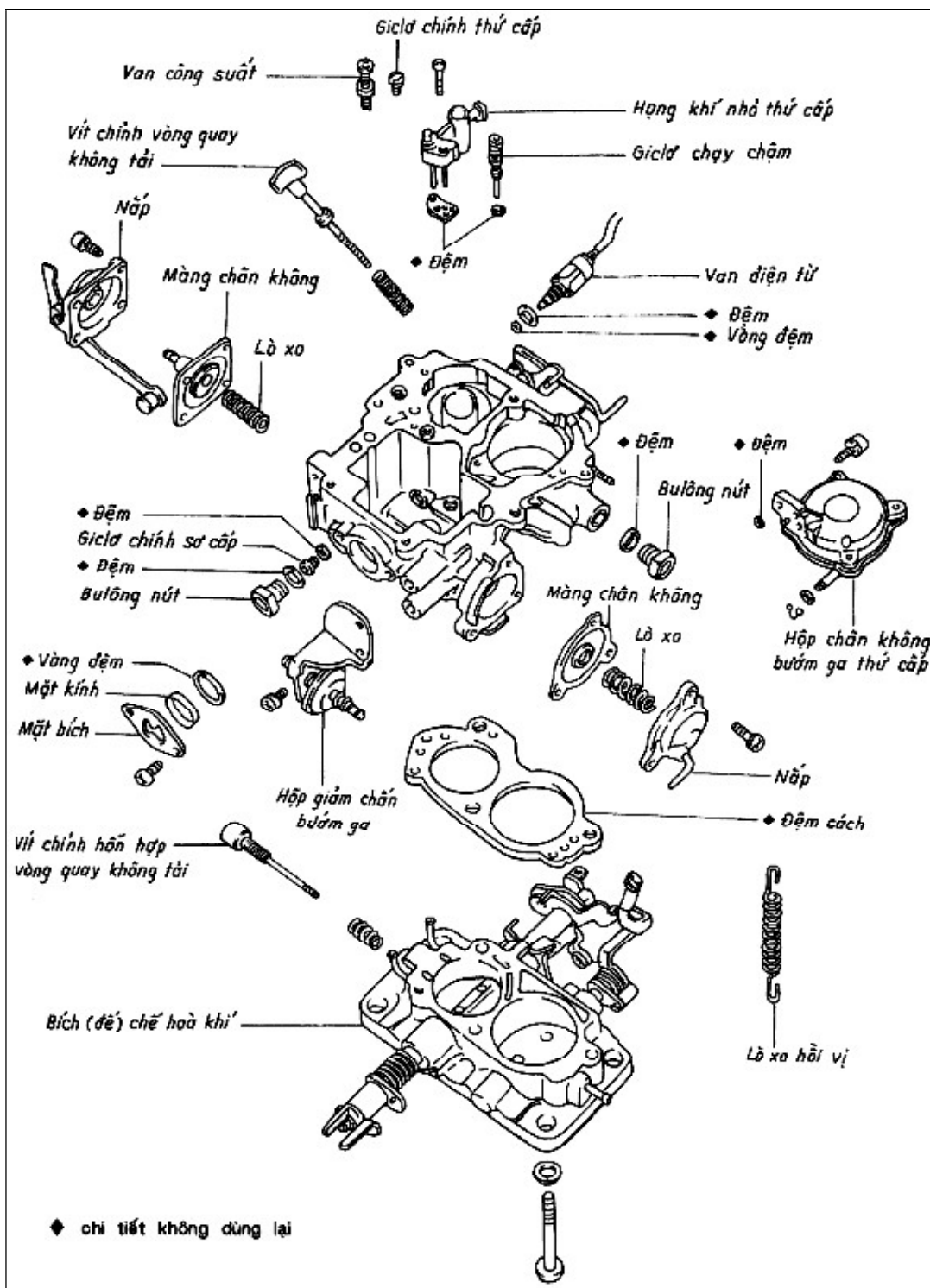
Hình 3.20. Tháo rời của thân và đế bộ chế hoà khí trên động cơ Toyota 1RZ, 2RZ
