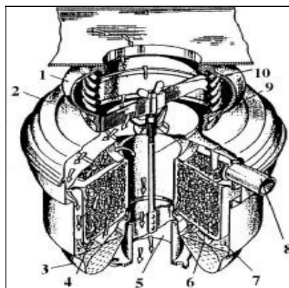
Hình 1.19. Bầu lọc không khí động cơ xăng.
