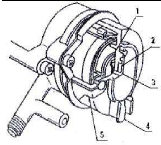
Hình 3.54. Cơ cấu điều khiển đóng mở bướm ga bằng điện
