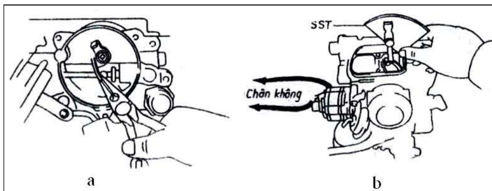
Hình 3.30. Kiểm tra góc mở bướm gió
