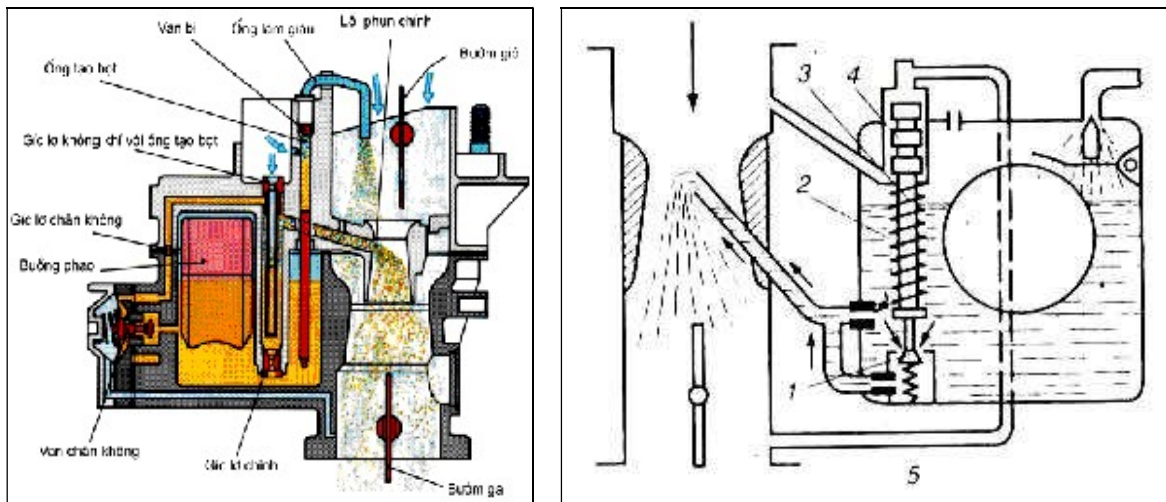
Hình 3.47. Cơ cấu làm đậm
