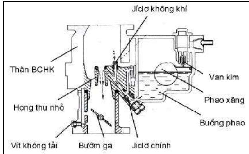
Hình 1.22. Sơ đồ cấu tạo bơm xăng và bộ chế hoà khí
