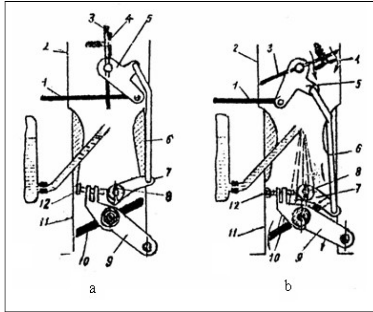
Hình 3.4. Cơ cấu khởi động
