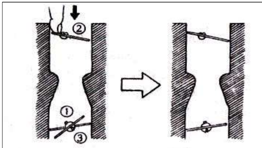
Hình 3.27. Điều chỉnh cơ cấu chân không
