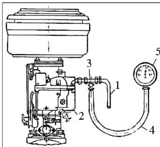
Hình 5.2. Kiểm tra áp suất bơm xăng
