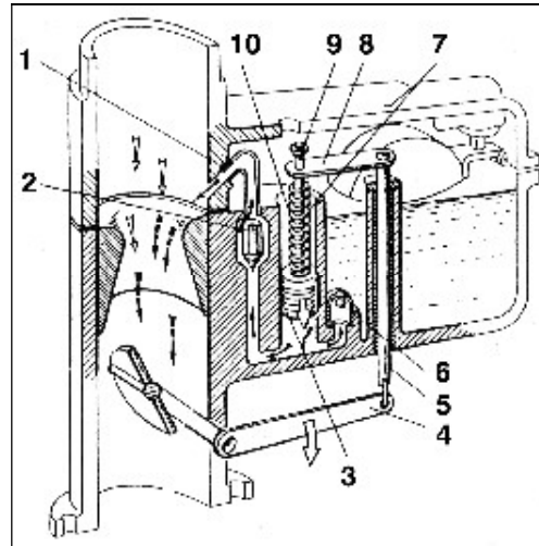
Hình 3.8. Hệ thống tăng tốc
