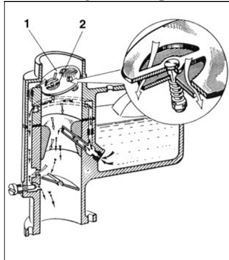
Hình 3.3. Hệ thống khởi động 1. Bướm gió; 2. Van khí phụ
